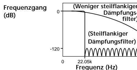
Vergleich der Grenzfrequenzcharakteristik von steifflankigen und weniger steifflankigen Dämpfungsfilern
