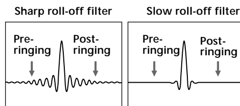
Vergelijking tussen de impulsrespons van een sharp roll-off filter en een slow roll-off filter
