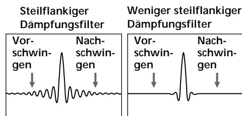
Vergleich der Impulsantwort von steifflankigen und weniger steifflankigen Dämpfungsfilern
