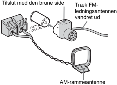
AM-rammeantenne
