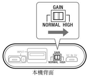
本機背面
