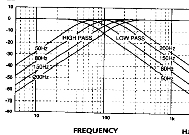
Cut-off frequency/Fréquence de coupure dB
