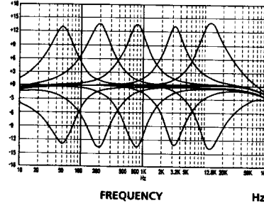
Cut-off frequency/Fréquence de coupure dB
