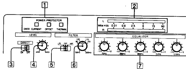
Equalizer/Egaliseur dB
